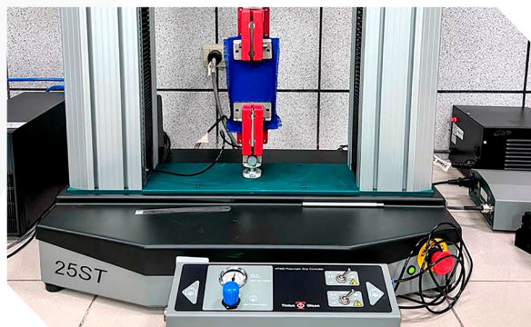
Dinamómetro 20kN
